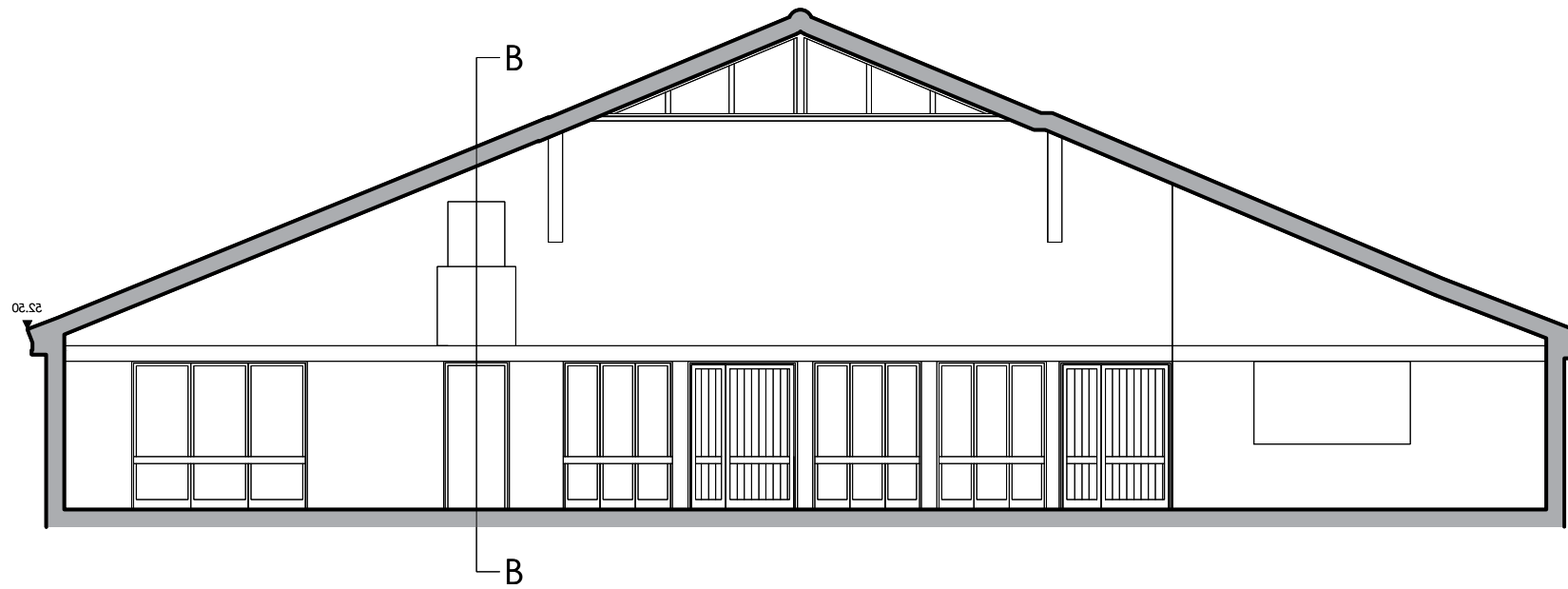
Existing Section A-A 1:100
